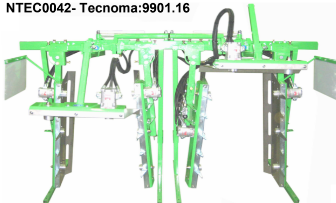
VUE AVANT DE LA MACHINE
