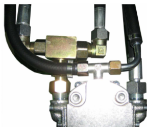
DETAIL VANNE 3 VOIES
